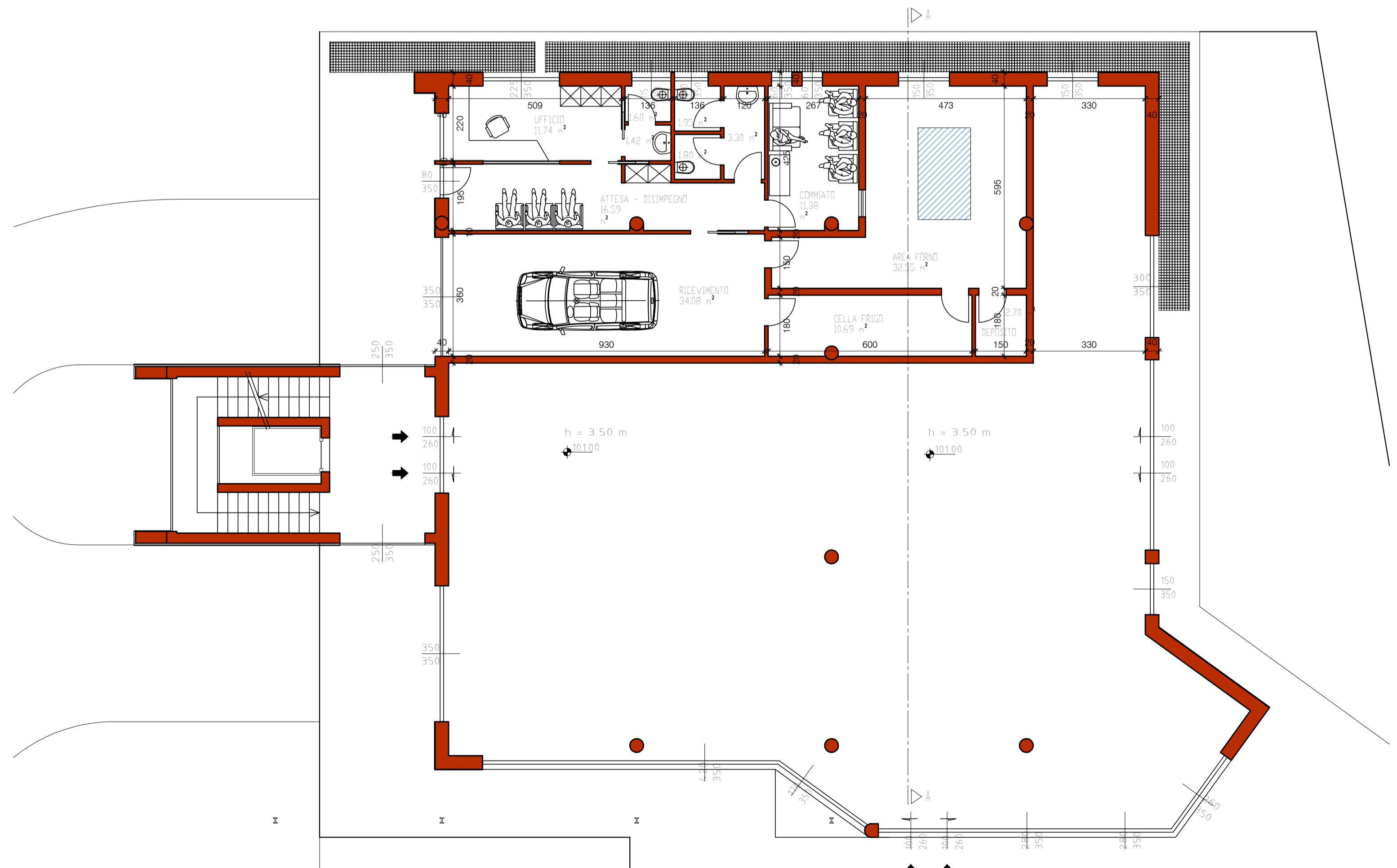
Pianta scala 1:100
